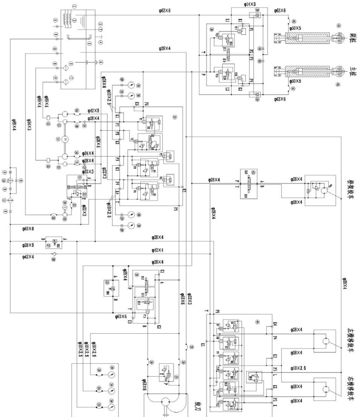
120m 3 /h 绞吸式挖泥船液压系统原理图
